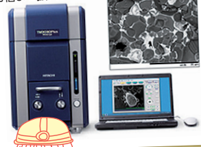
走査型電子顕微鏡(HITACHI TM3030Plus) 1万倍まで拡大してチェック!
